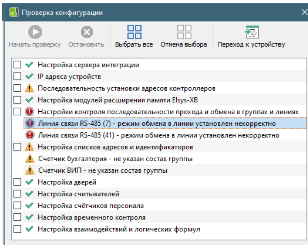
Рис. 14 Форма проверки конфигурации системы
