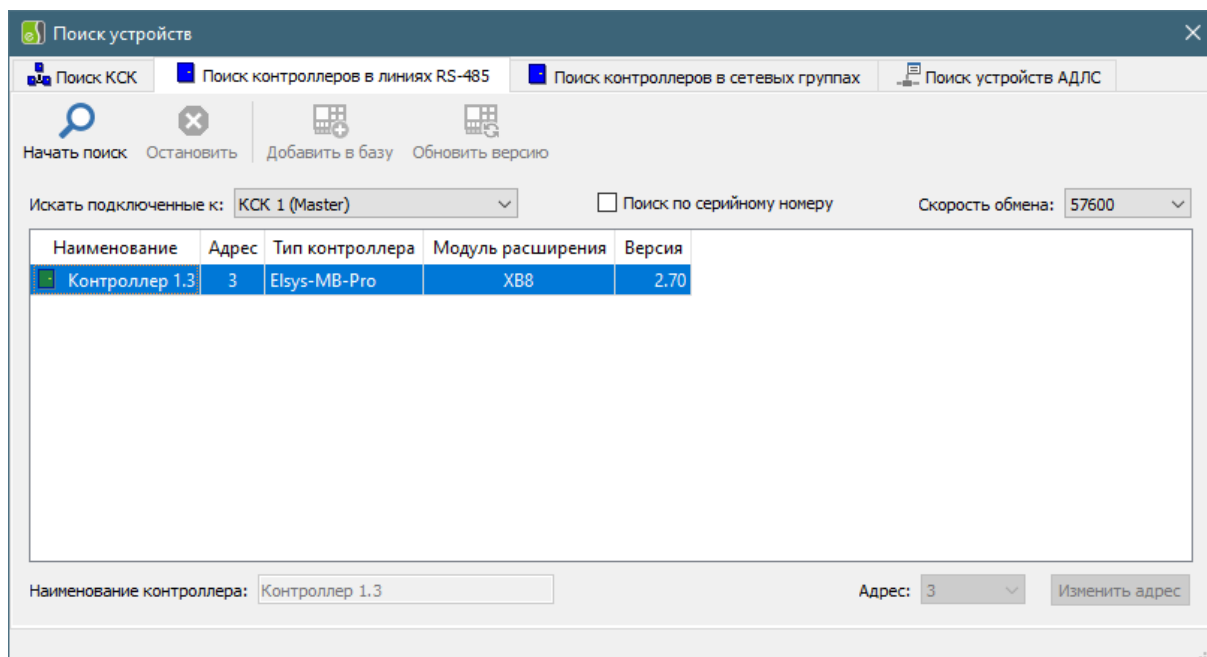
Рис. 7 Окно формы поиска контроллеров с интерфейсом RS-485
