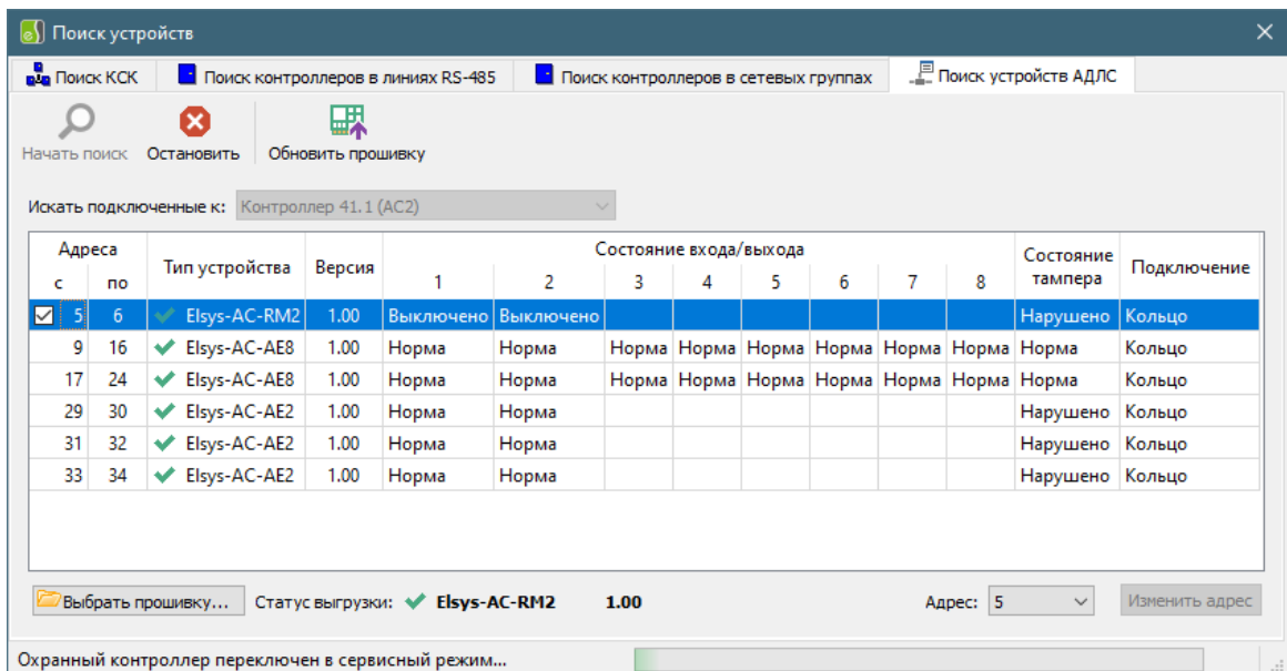
Рис. 9 Окно формы поиска и конфигурирования устройств АДЛС
