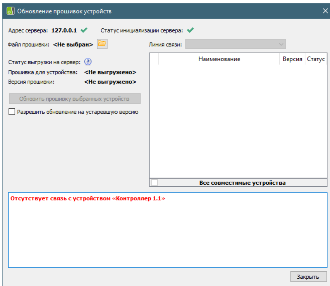
Рис. 18 Форма управления процессом обновления прошивок устройств
