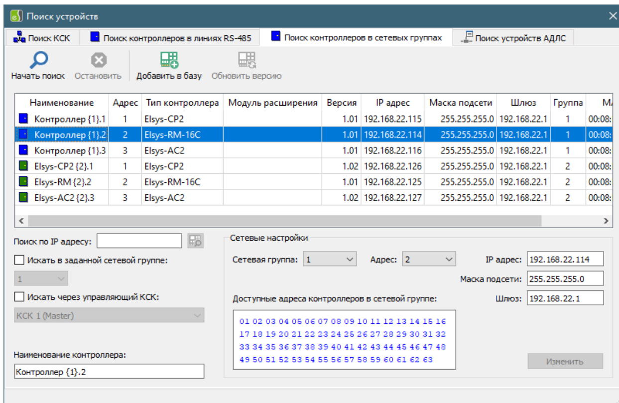
Рис. 8 Окно формы поиска контроллеров с интерфейсом Ethernet
