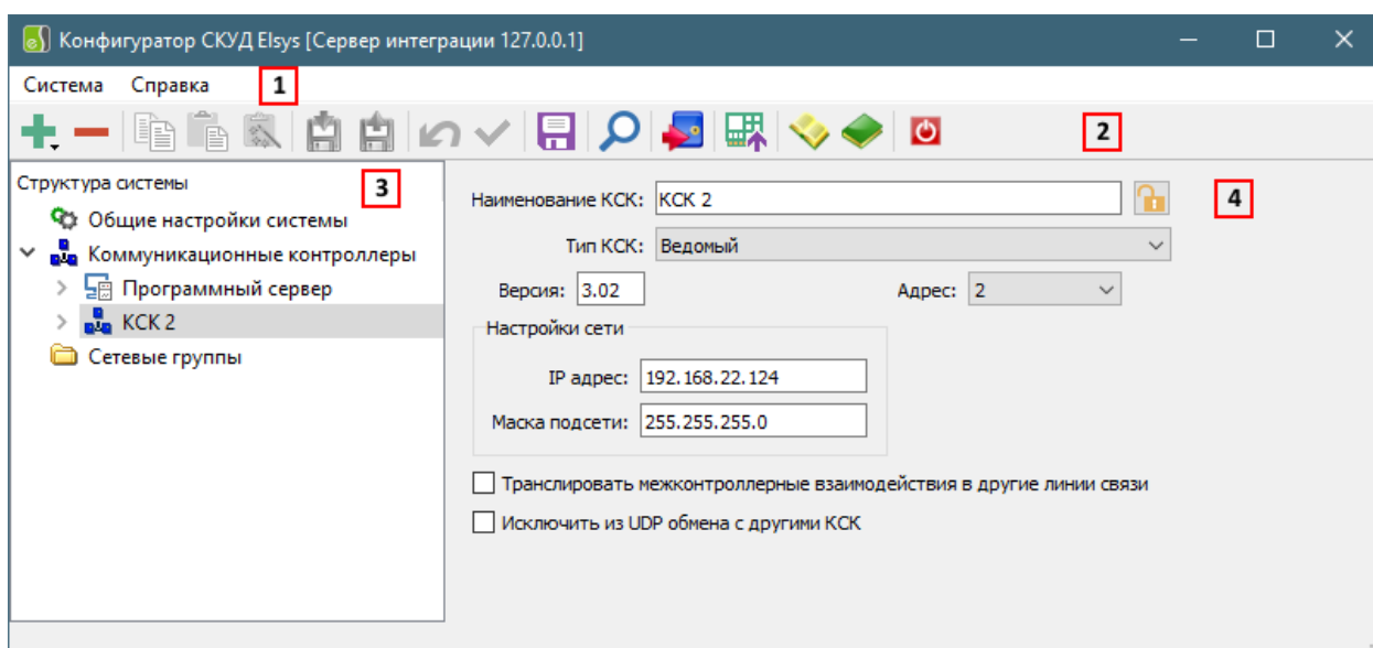
Рис. 4 Пользовательский интерфейс приложения
