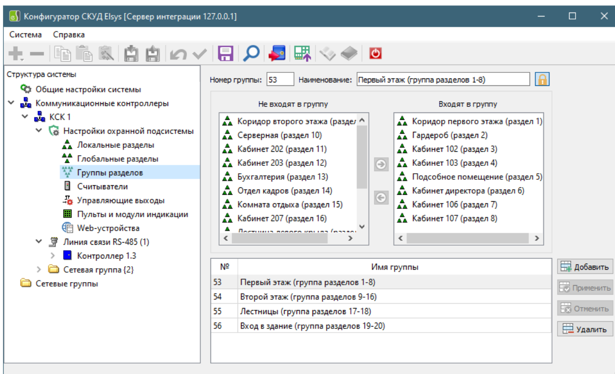
Рис. 13 Панель настройки параметров группы разделов
