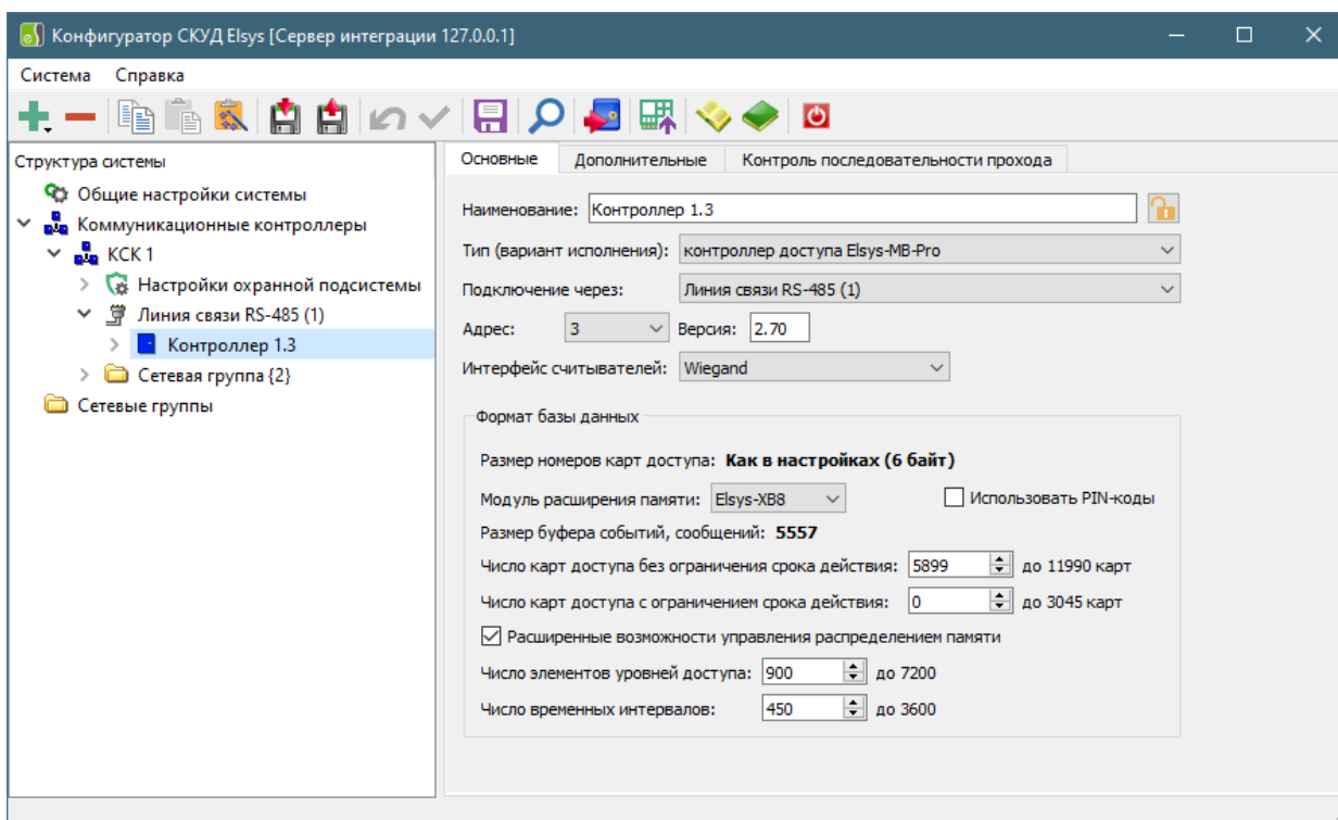
Рис. 12 Панель настройки параметров контроллера
