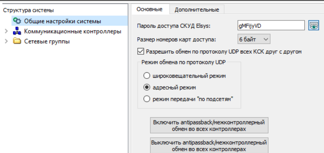
Рис. 16 Вкладка настройки общих параметров системы
